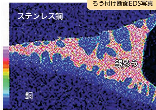
ろう付け断面EDS写真
